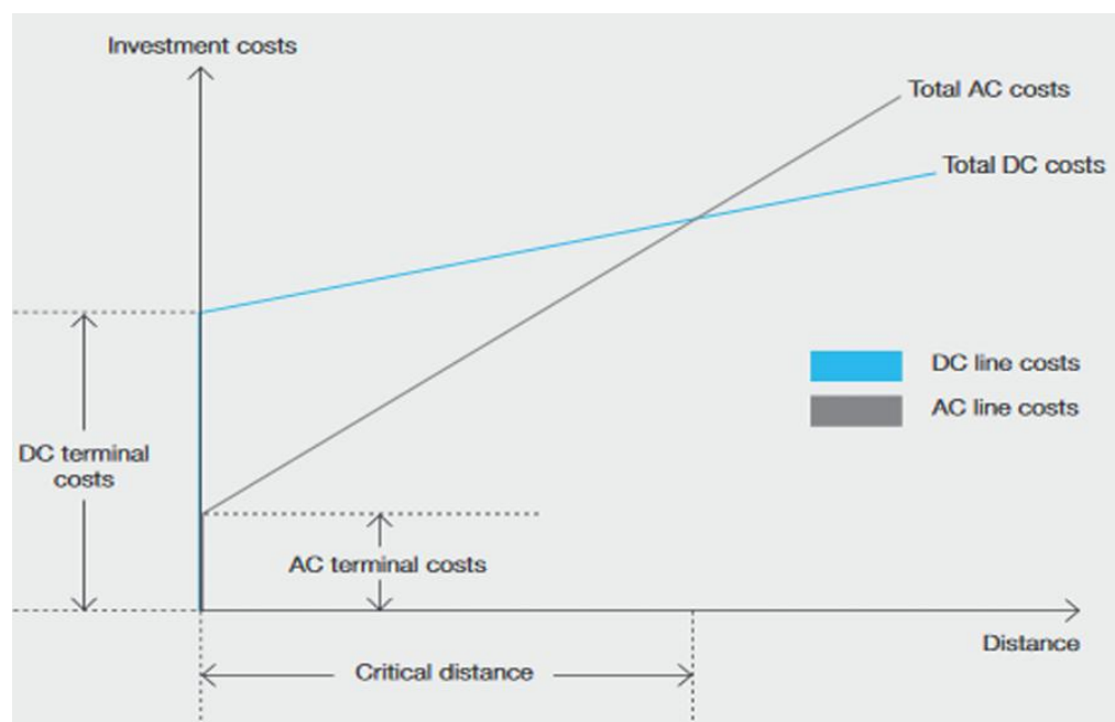
Figure 28. AV and HVDC Breakeven Cost Illustration 136
