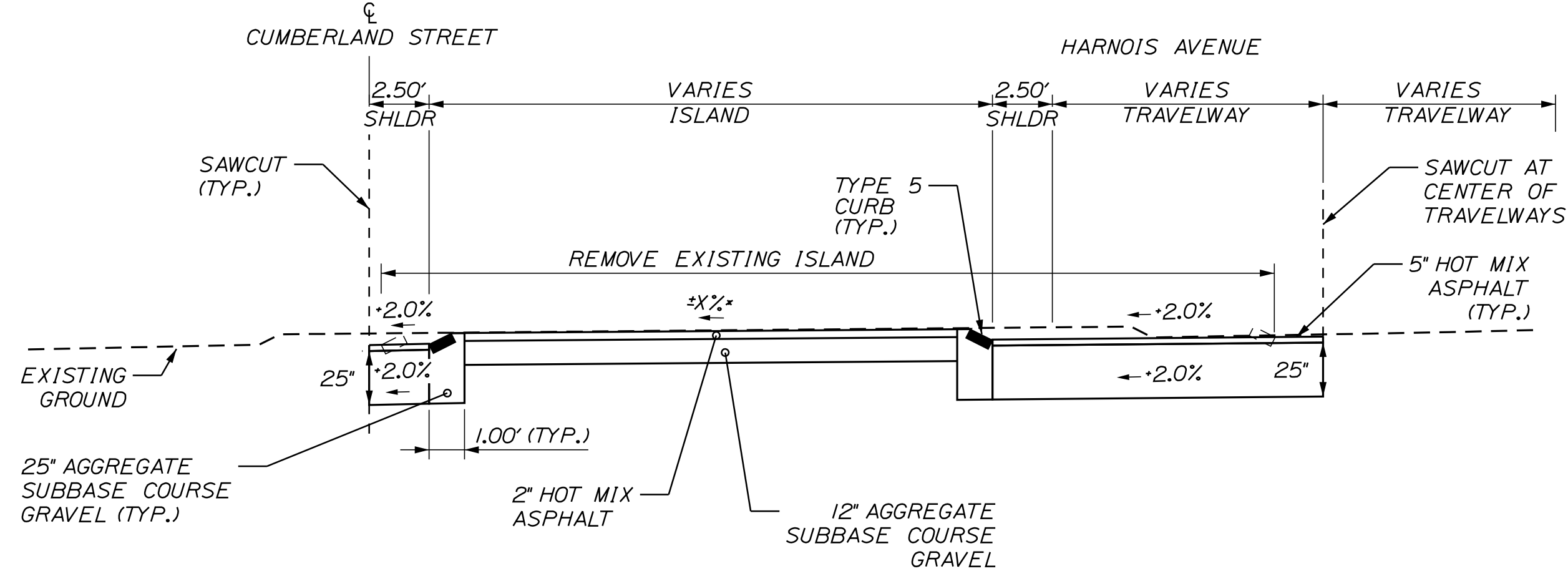
CUMBERLAND STREET & HARNOIS AVENUE DETAIL G-G (N.T.S.)
