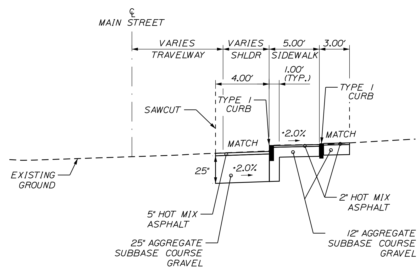
SHOULDER RECONSTRUCTION - CURB TYPE 1 STA. 32+76 TO 33+00 RT (N.T.S.)
