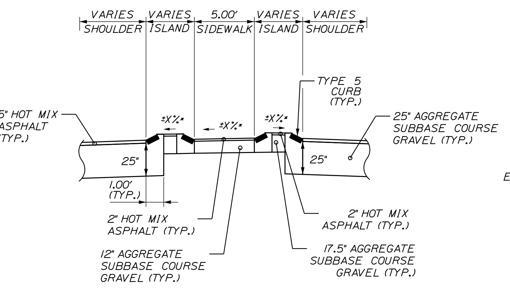
INTERIOR ISLAND DETAIL (N.T.S.)
