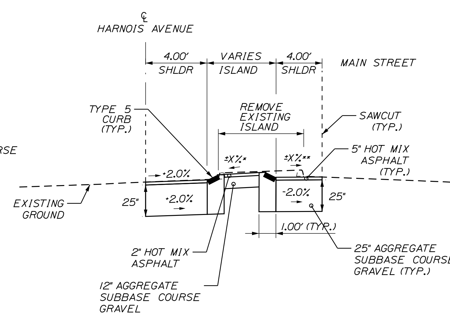
HARNOIS AVENUE & MAIN STREET DETAIL A-A (N.T.S.)
