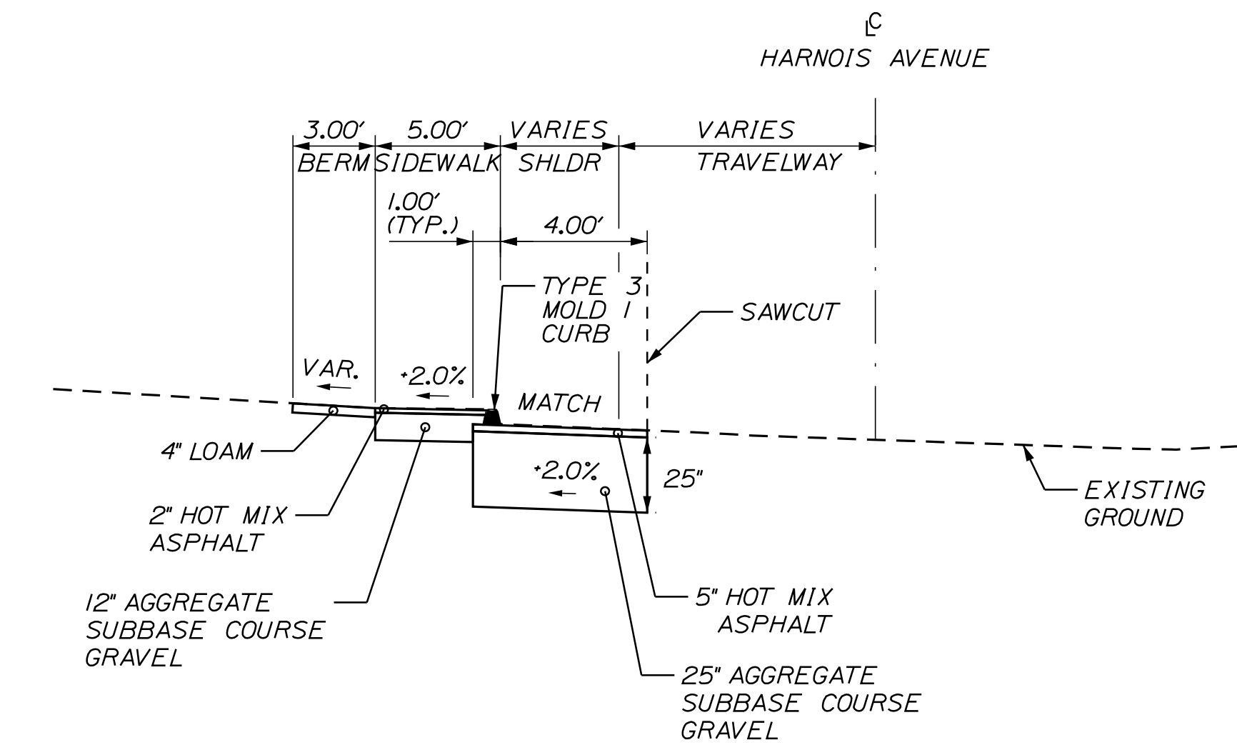
SHOULDER RECONSTRUCTION - CURB TYPE 3 STA. 66+60 TO 66+93 LT (N.T.S.)
