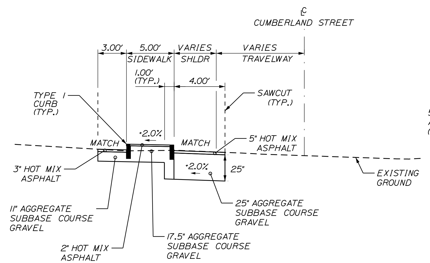
SHOULDER RECONSTRUCTION - CURB TYPE 1 STA. 14+44 TO 14+67 LT (N.T.S.)
