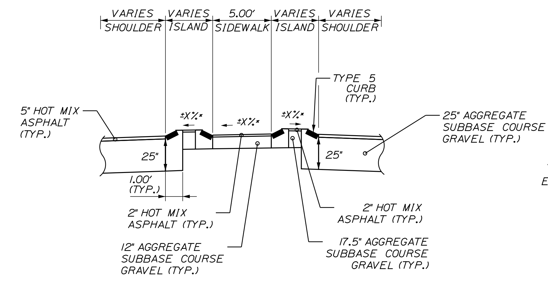
INTERIOR ISLAND DETAIL (N.T.S.)
