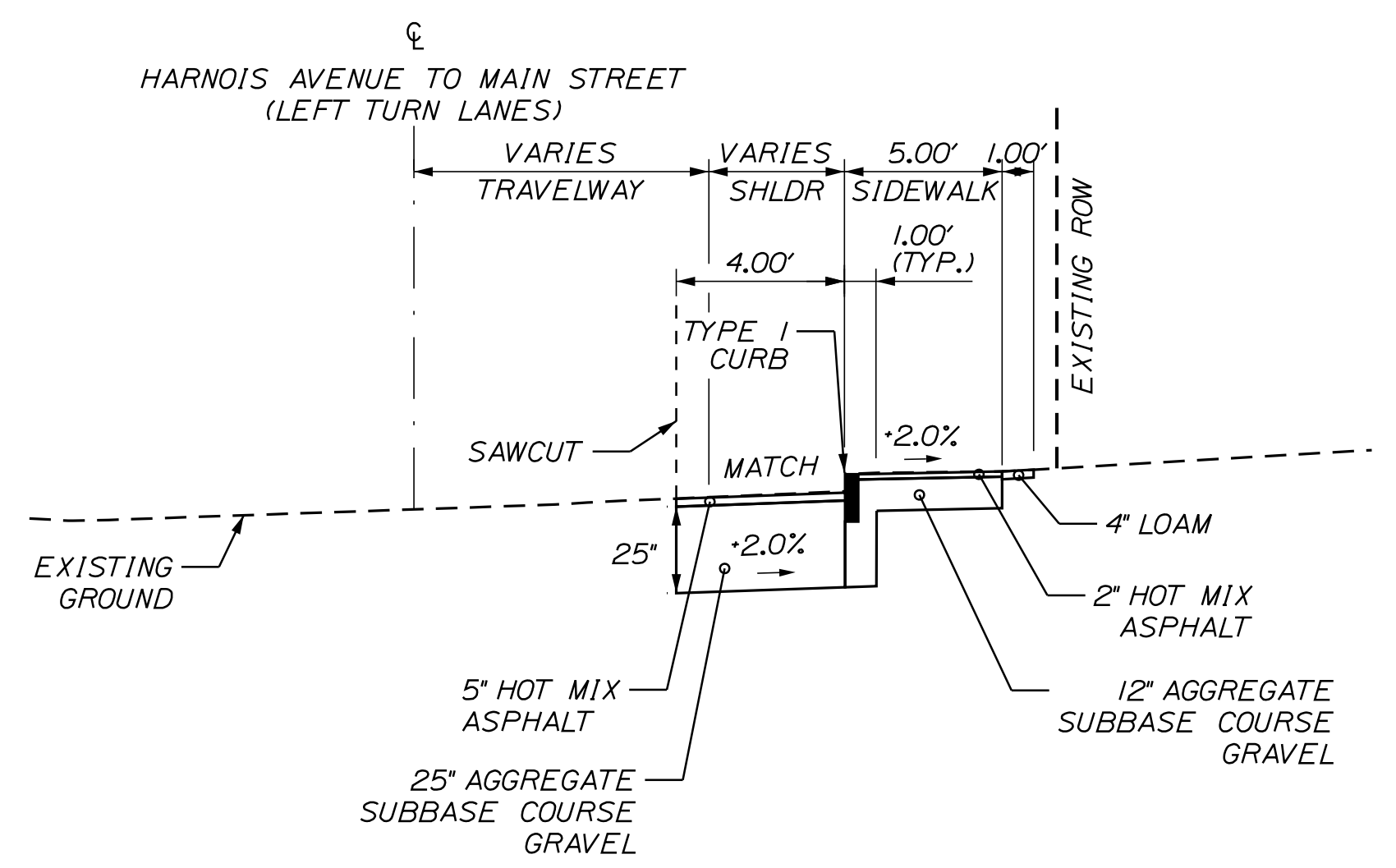
SHOULDER RECONSTRUCTION - CURB TYPE 1 STA. 73+95 TO 74+65 RT (N.T.S.)
