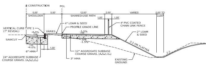
SHARED USE PATH STA. 102+75.00 TO STA. 110+50.00 STA. 116+25.00 TO STA. 117+75.00
