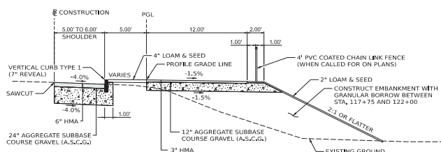
SHARED USE PATH STA. 100+50.00 TO STA. 101+50.00 STA. 110+50.00 TO STA. 112+00.00 STA. 117+75.00 TO STA. 122+25.00
