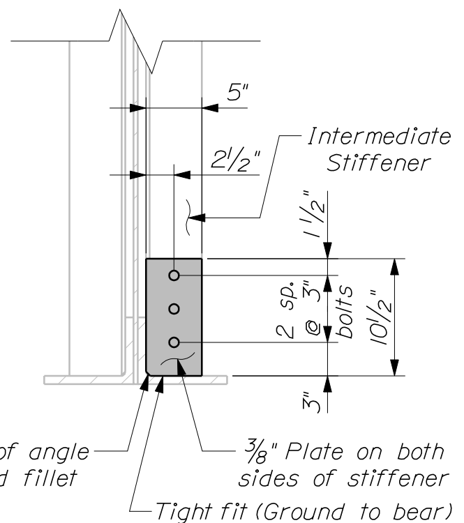
SECTION A-A
